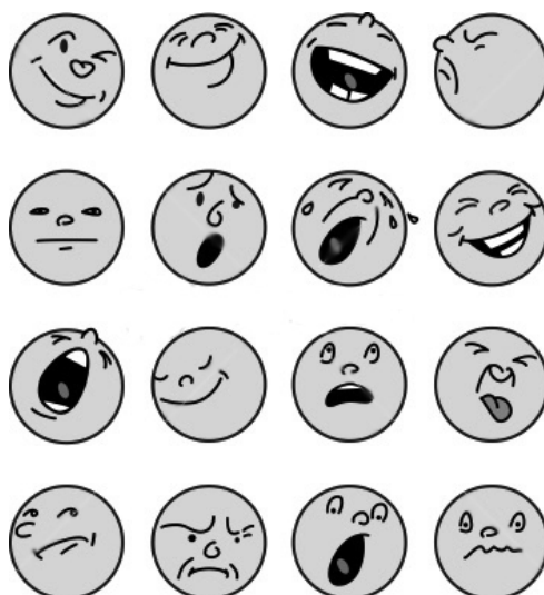
شکل ۲- ۸ دیکشنری احساسات
