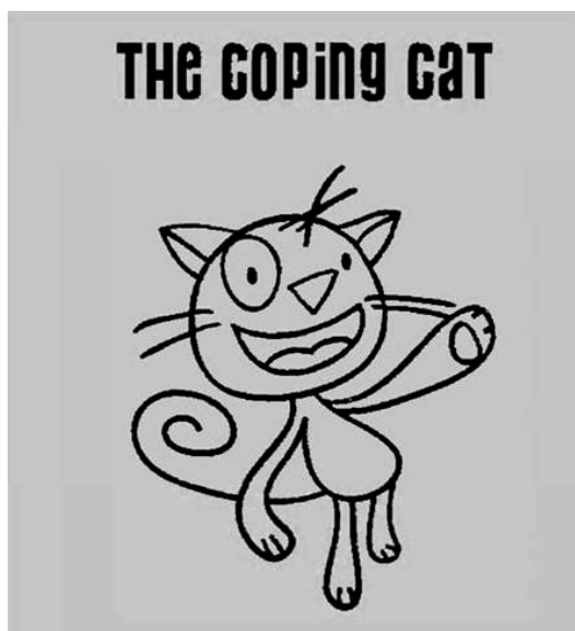
شکل ۸-۱ گربه ی سازشگر
